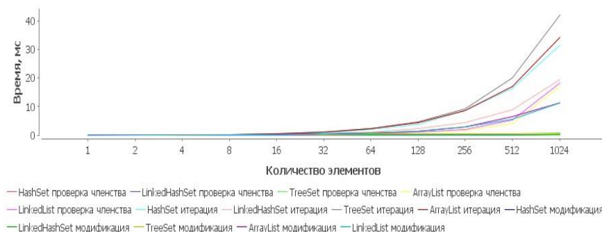
Рис. 1. Сравнение производительности коллекций на небольшом наборе данных
